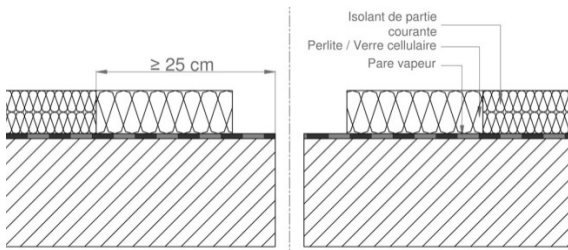
Figure 14 – Terrasses accessibles aux piétons et séjour - Feuillure sur support isolant rapporté
