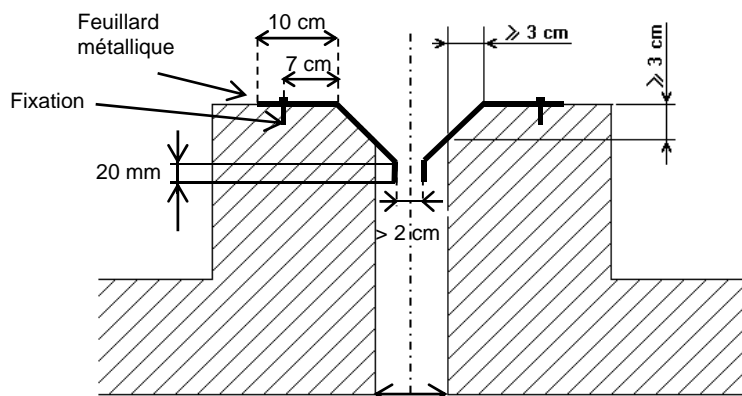
Figure 4 – Exemple de traitement d'un joint sur costière en zone de sismicité concernée par la réglementation
