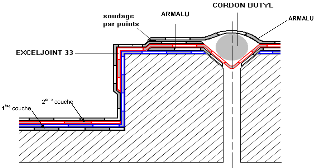
Figure 16 – Exemple de traitement d'un joint sur costière
