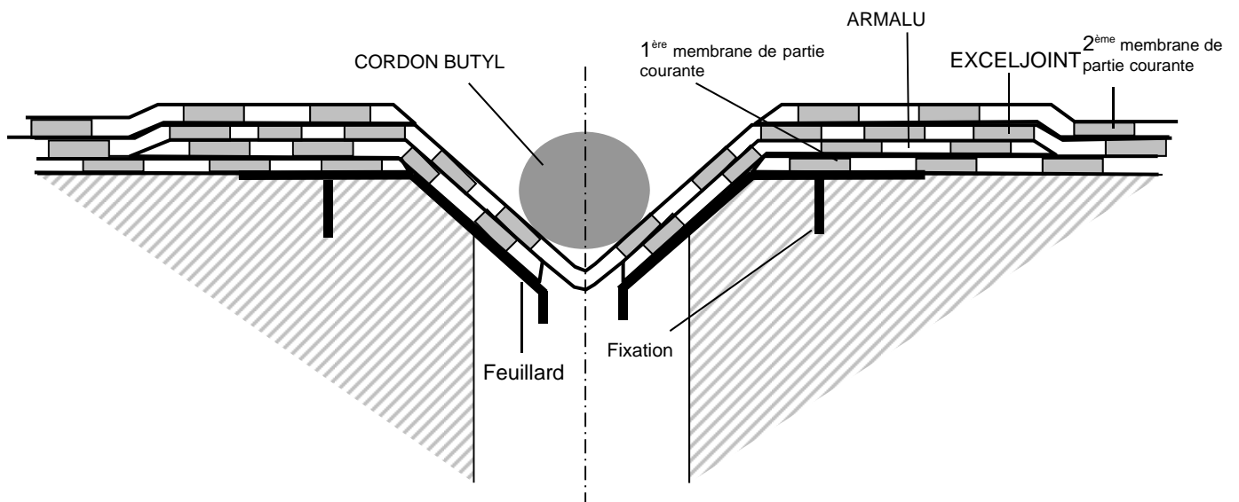
Figure 20 – Joint en zone de sismicité concernée par la réglementation (détail de mise en œuvre)
