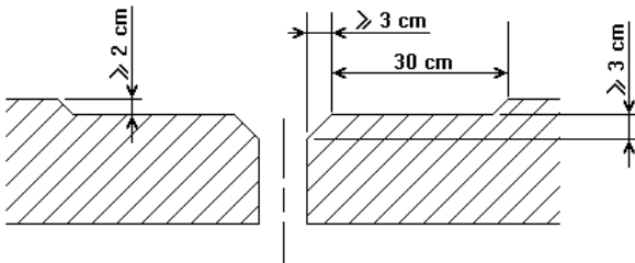
Figure 9 – Feuilleure pour étanchéité asphalte
