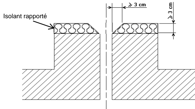
Figure 3 – Costière avec forme de chanfrein (perlite expansée ou verre cellulaire)
