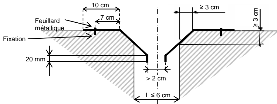
Figure 8 – Joint en zone de sismicité concernée par la réglementation
