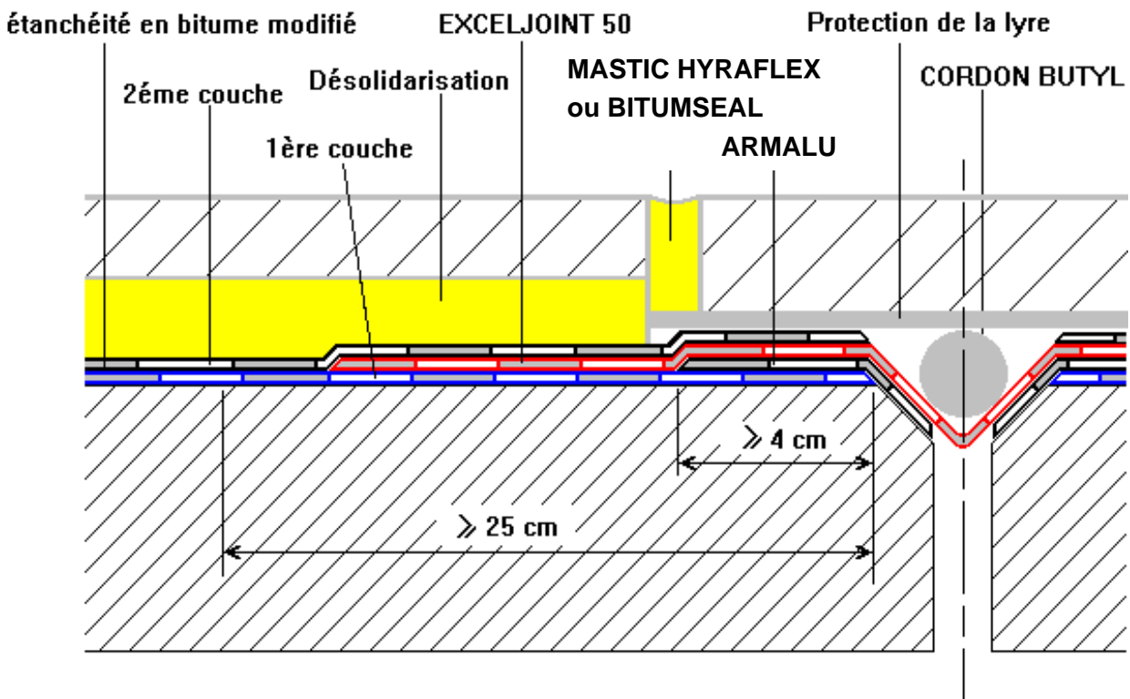
Figure 17 – Joint plat en partie courante raccordé à une étanchéité en bitume modifié, en terrasse accessible aux piétons
