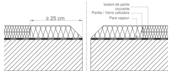
Figure 13 – Terrasses accessibles aux piétons et séjour - chanfreins sur support isolant rapporté
