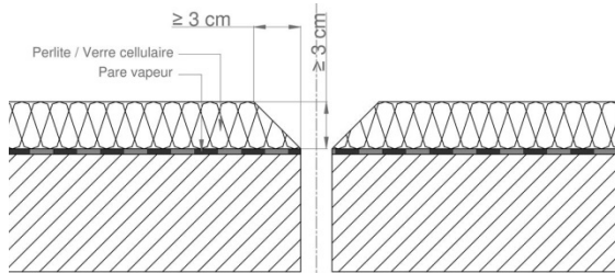
Figure 12 – Terrasses accessibles aux piétons et séjour – chanfreins sur isolants perlite expansée ou verre cellulaire
