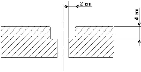
Figure 6 – Feuille dans les supports en béton
